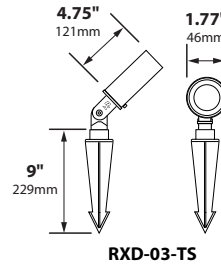
RXD-03-TS
