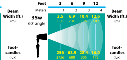
FL-15-FMV-FG FL-15-FMV-ULTRA
