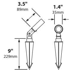
RXD-04-TS
