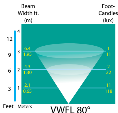
FL-LED-MR16SS5W80
