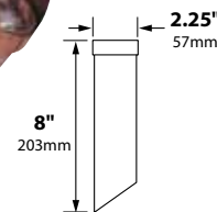
SL-36-MR16
