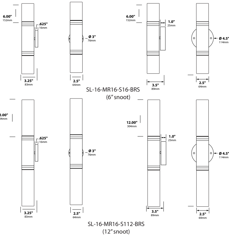
SL-16-MR16-S16-BRS (6" snoot)
