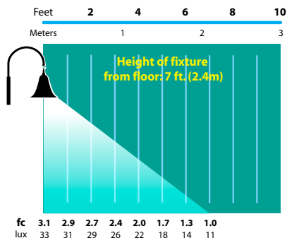
SL-05-WM
