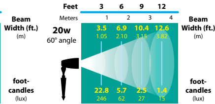
FL-13-VWFL-FG
