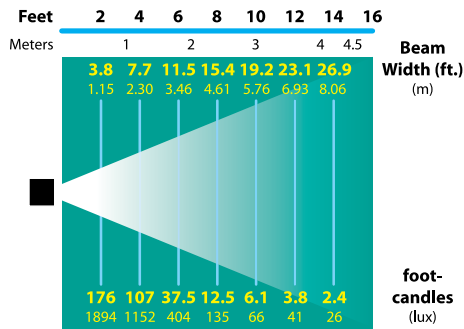
35w T-4 DC Halogen
