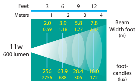
DL-43-LEDM1140 40° FLOOD
