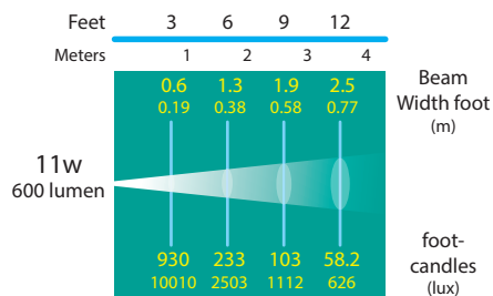
DL-43-LEDM1115 15° SPOT
